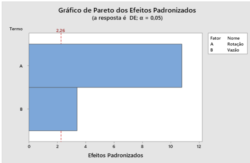
Figura 4 – Influência da rotação e da vazão no dado colorimétrico \Delta E
